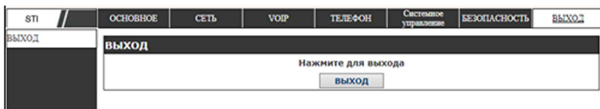
Рисунок 57 – Выход
