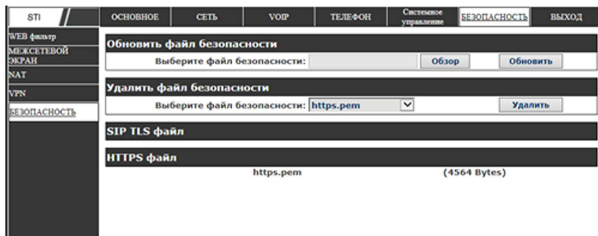
Рисунок 2.56 – Безопасность
