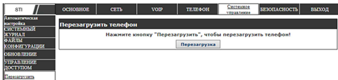
Рисунок 2.51 – Перезагрузить
