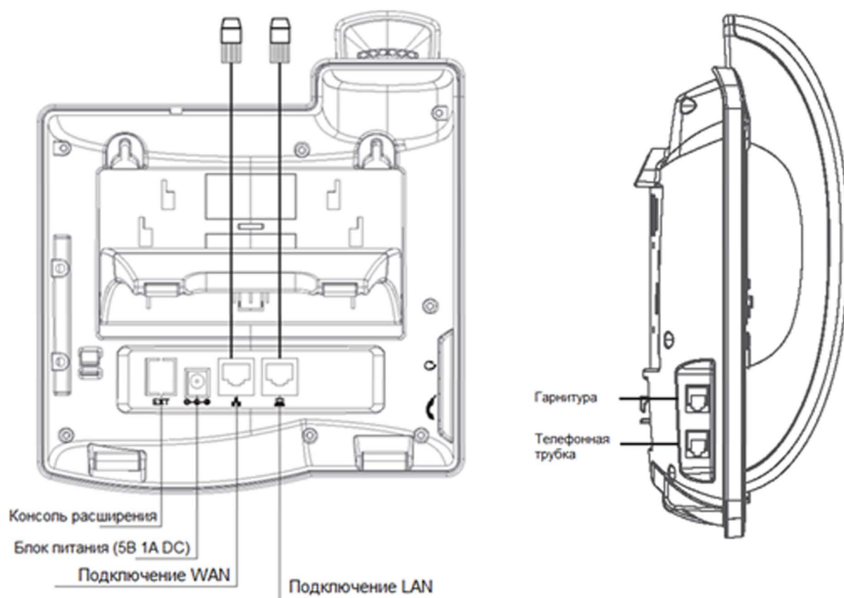
Рисунок 1.2 – Расположение портов подключения изделия
