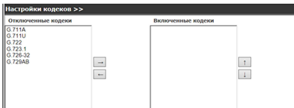
Рисунок 2.28 – Настройки кодеков
