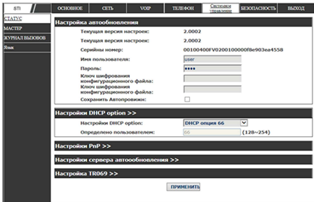
Рисунок 2.41 – Статус
