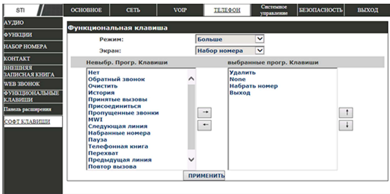
Рисунок 2.40 – Софт-клавиши
