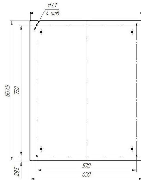
Рисунок 2 – Установочные размеры контроллера ТБС-ВК
