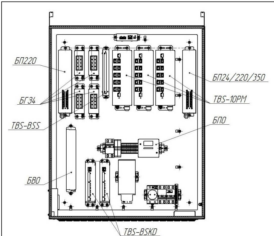
Рисунок 1 – Размещение блоков на монтажной панели
