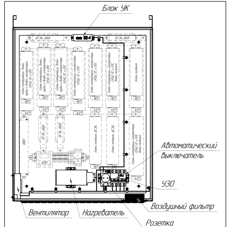
Рисунок 1 – Размещение блоков на монтажной панели (расположение элементов может отличаться от приведенного)
