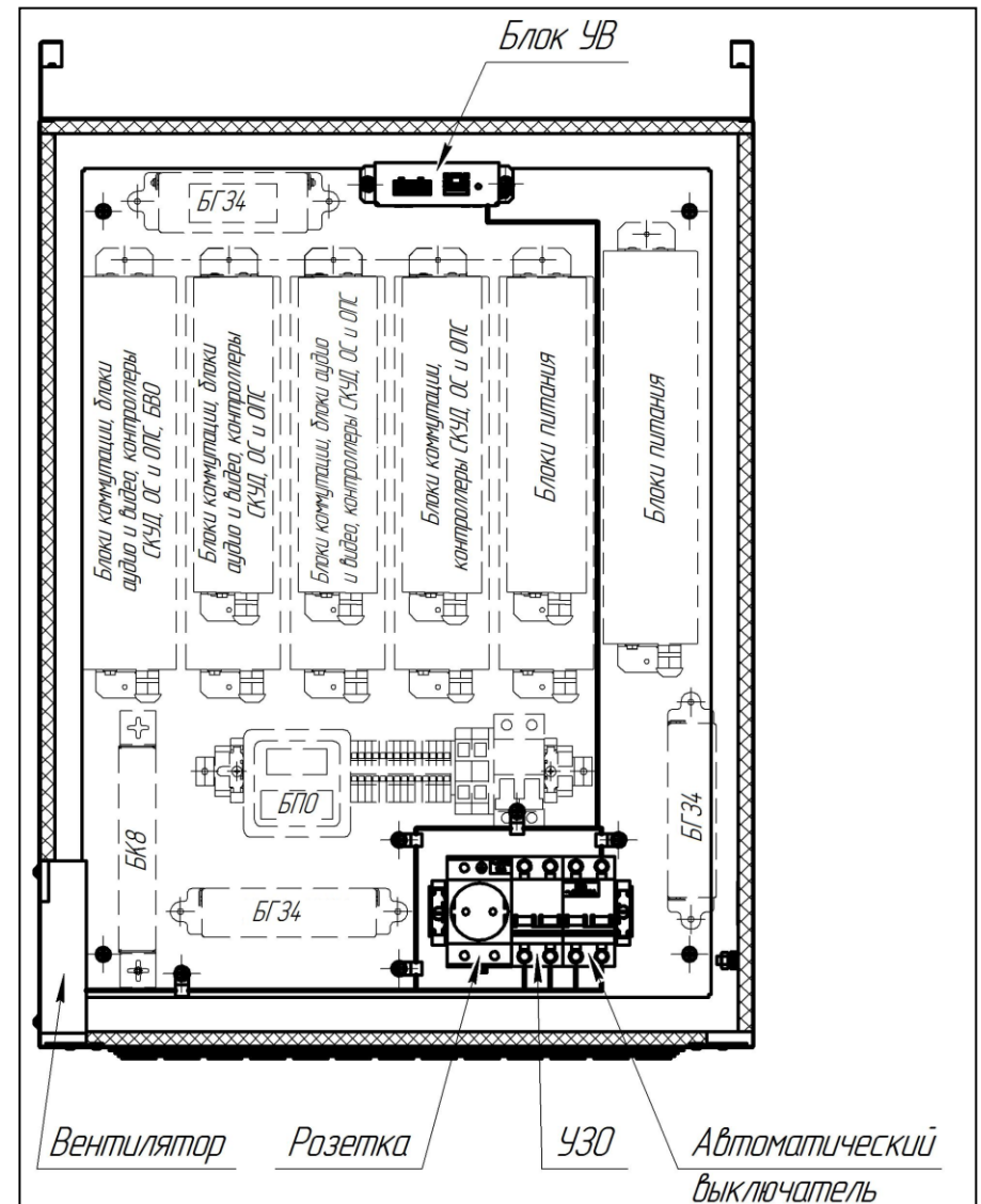
Рисунок 1 – Размещение блоков на монтажной панели
