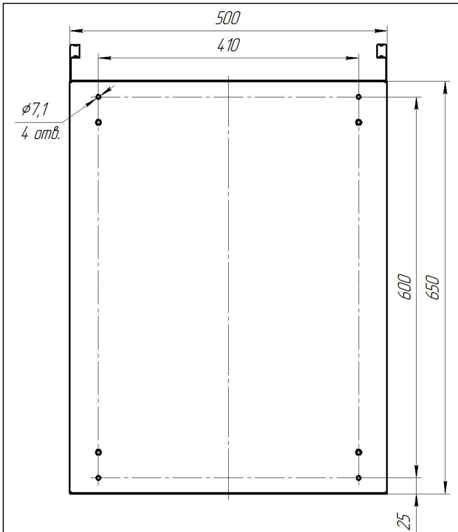
Рисунок 2 – Установочные размеры контроллера STS-504А
