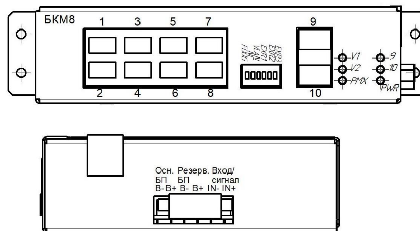
Рисунок 1 – Назначение разъемов коммутатора БКМ8.
