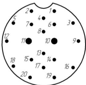
Рисунок 1 – Обозначение контактов разъема (вилка).
