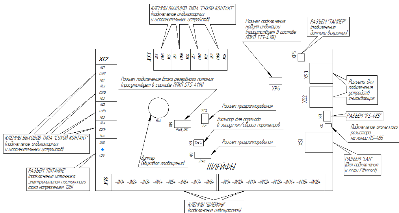
Рисунок 3 – Назначение разъемов платы контроллера ОС TBS-SS
