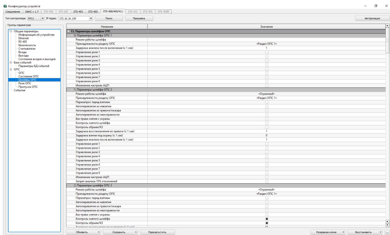
Рисунок 26 – Шлейфы ОПС
