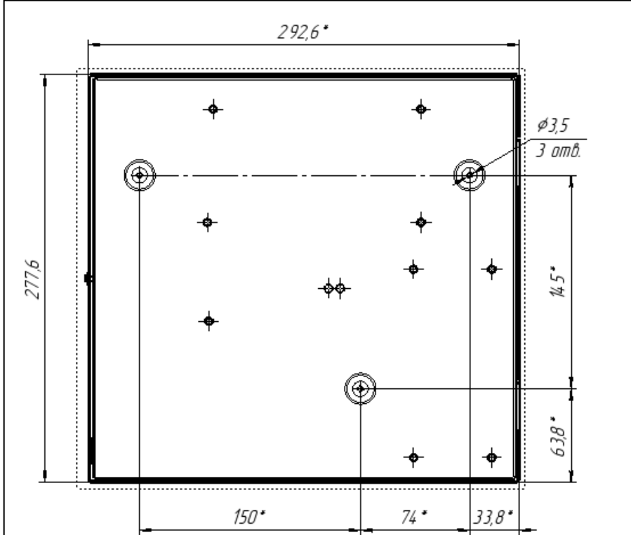
Рисунок 3 – Установочные размеры контроллера СТС-408К
