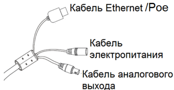
Рисунок 1 – Подключение видеокamеры
