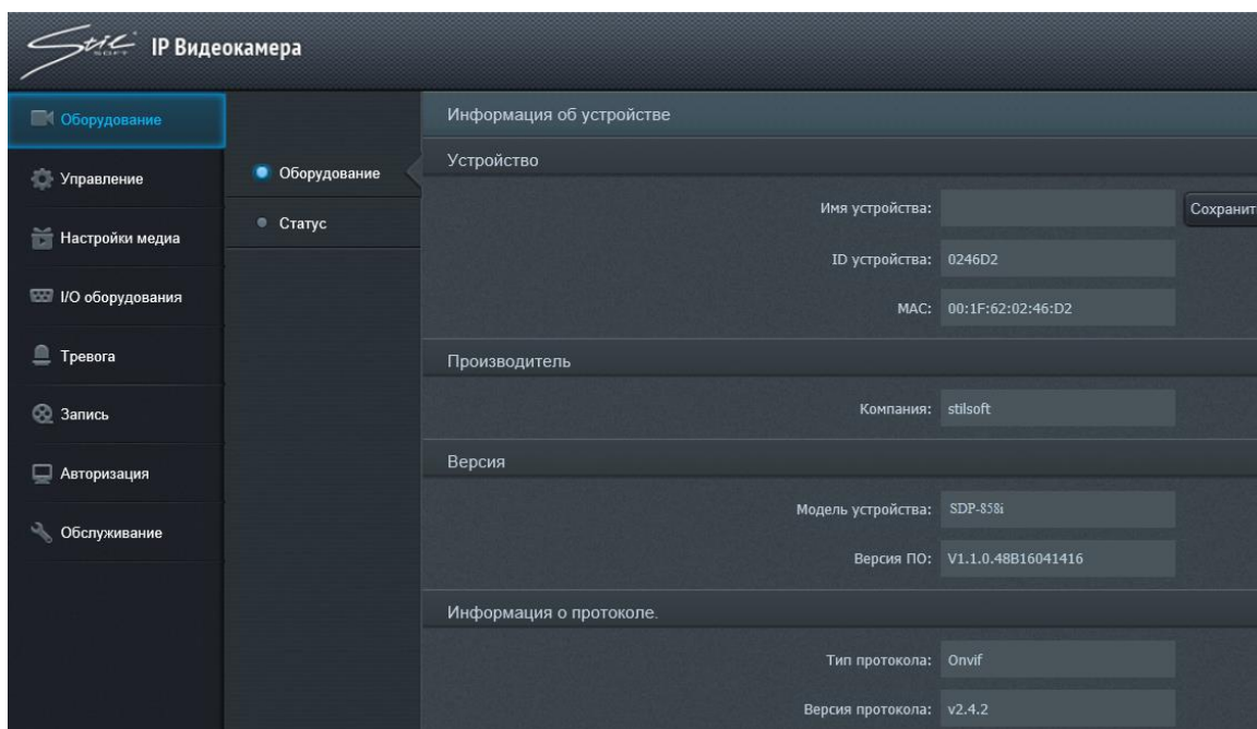
Рисунок 7 – Меню настроек видеокамеры
