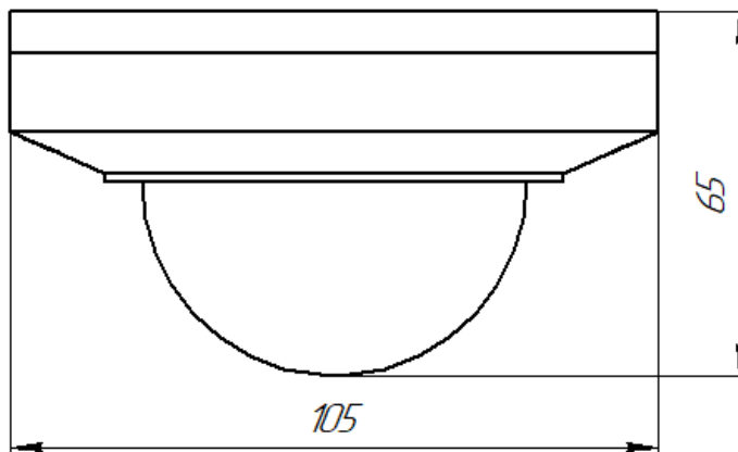
Рисунок 2 – Габаритные размеры IP-видеокамеры SDP-859
